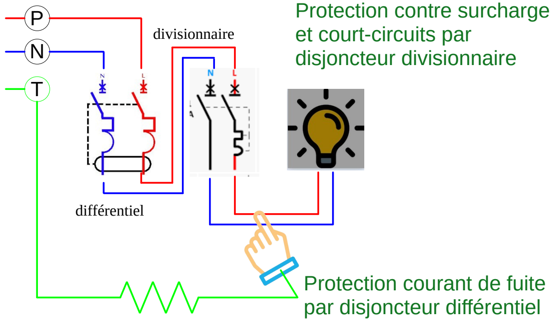
Disjoncteur divisionnaire
